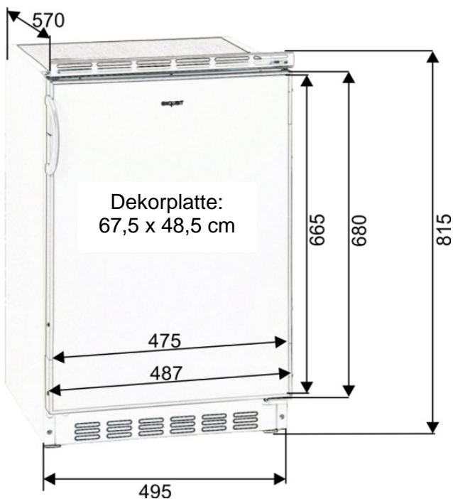
Unterbau-skizze
