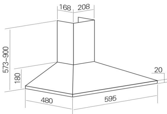
Einbauskeizze
