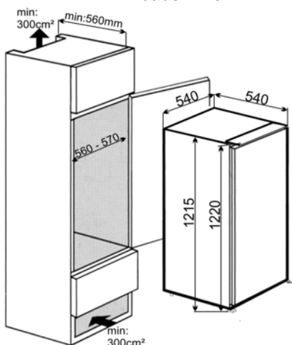
Einbauskizze
